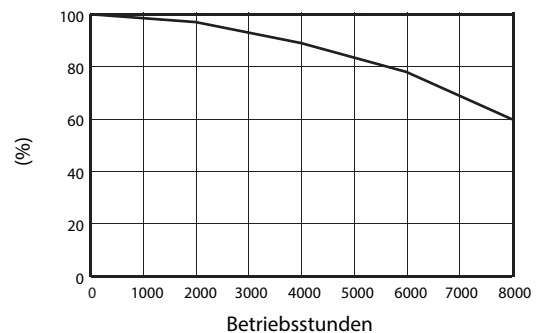
Lampen-Lebensdauer
