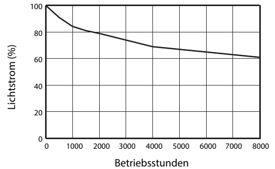
Lichtstromverhalten
